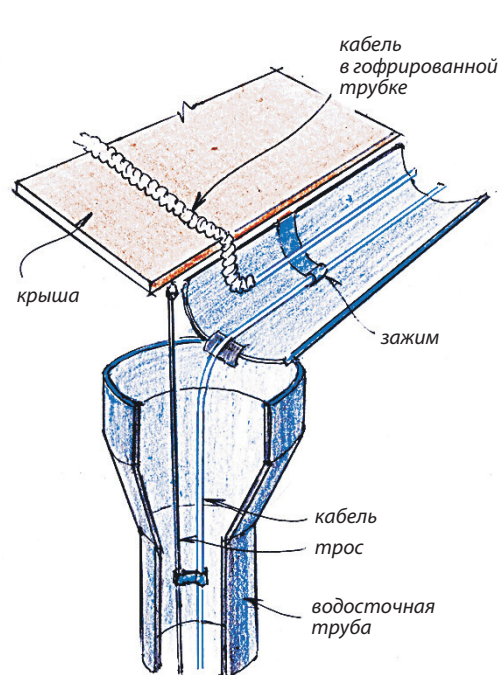
Рис. 1 Кабель в водостоке
