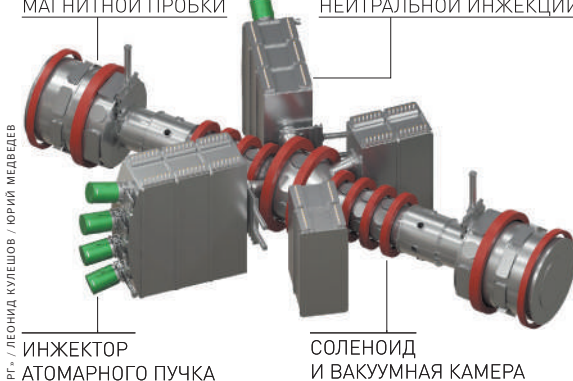
В инжекторе генерируются атомы, которые разогревают плазму. В камере нейтральной инжекции они очищаются от «вредных» ионов. Сверхпроводящие магниты удерживают плазму в «трубе». Температура плазмы должна достигать 150 миллионов градусов.
